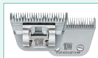
GT339 (#10W) 5/64" | 2,4 mm
